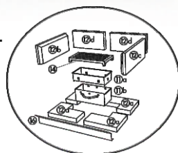
Feuerraum Aufbau
