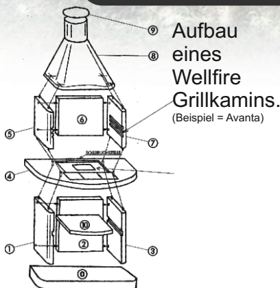
Feuerraum Aufbau
